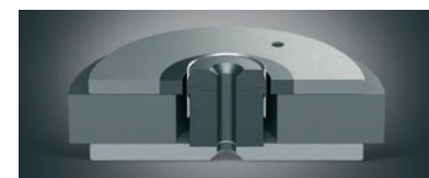
SMC マグネットシステム (磁気回路)
